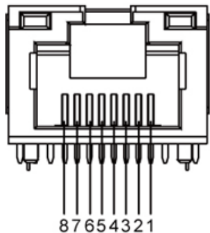
RJ45-Ausgang für 10BASE-T und 100BASE-TX
